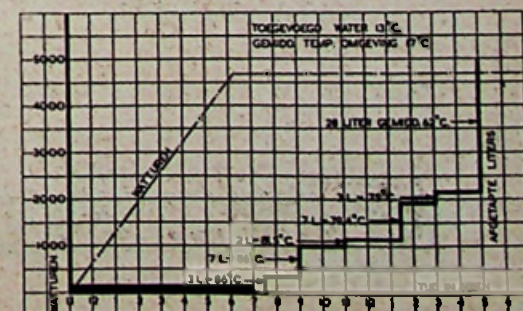
AANSLUITING EN AFTAPPIJNEN VAN EEN 30 LITER OVERLOOPRESERVOIR NACHTSTROOMTARIEF VAN 11-7 UUR. CAP VAN HET ELEMENT 600 WATT. THERMO SCHAKELAAR AFGESTELD TUSSEN 70-80°C.
