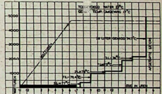
AANSLUITING EN AFTAPPIJNEN VAN EEN 30 LITER AFTAPRESERVOIR NACHTSTROOMTARIEF VAN 11-7 UUR. CAP VAN HET ELEMENT 600 WATT. THERMO SCHAKELAAR AFGESTELD TUSSEN 70-80°C.
