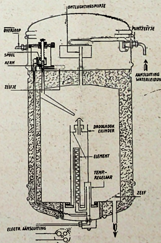
AANSLUITING EN AFTAPPIJNEN VAN EEN 30 LITER AFTAPRESERVOIR NACHTSTROOMTARIEF VAN 11-7 UUR. CAP VAN HET ELEMENT 600 WATT. THERMO SCHAKELAAR AFGESTELD TUSSEN 70-80°C.
