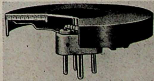
Een gedeeltelijk opengesneden kookplaat van Duits fabriikaat, ontleend aan Elektro-nwärme-Technik.
